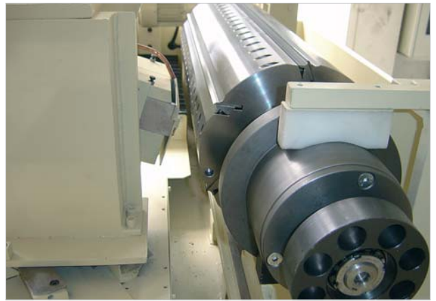
Hobelwelle, 670 mm, komplett mit Lagerungs-System und Steckkupplung in Schärffposition.
