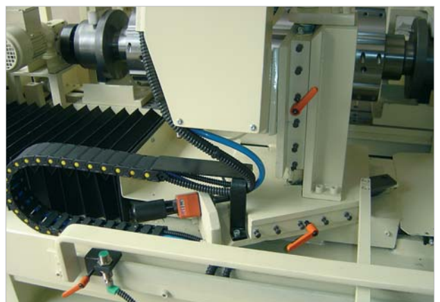
Umsetzbare Näherungsschalter zur Begrenzung des Fahrweges je nach Arbeitsbreite.
