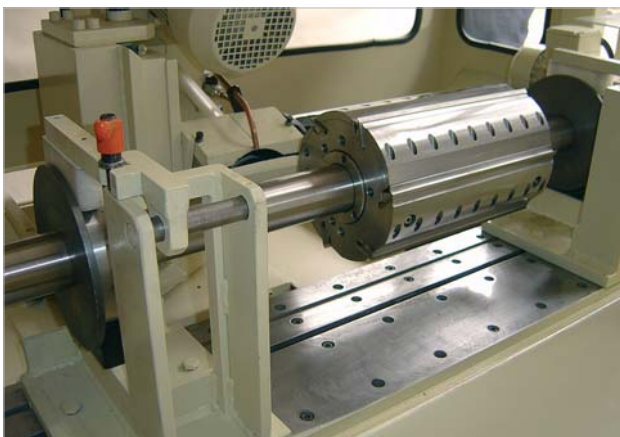
HydroKöpfe, 350 mm, mit Aufnahmewelle in Schärffposition.
