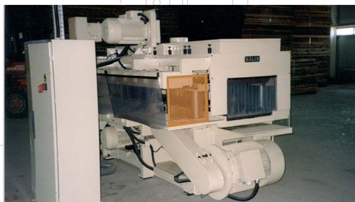
2-seitige Breithobelmaschine mit angebauter Vielblattsäge «INDUSTRY-HQ» 2MS
