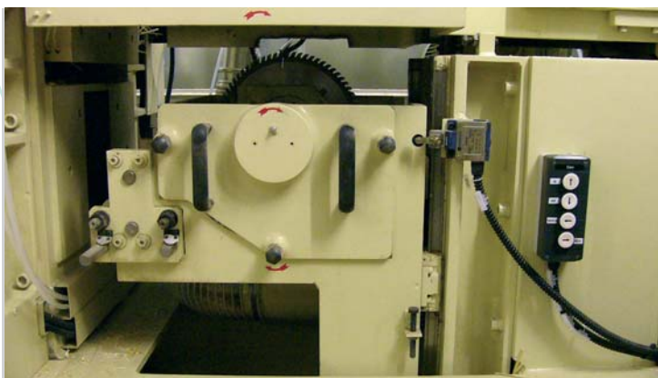
Ritzaggregat am Maschinen-Einlauf zum wechselseitigen Nuten von Breitlamellen
