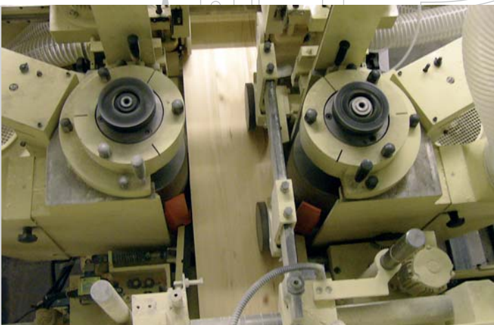
Vertikaleinheiten mit herausnehmbaren Hobelwellen (beidseitig einsetzbar)
